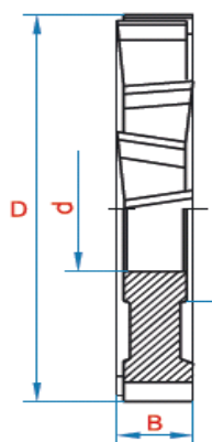
DIN8047 - Фрези дискови тристранни със запоени твърдосплавни пластини
